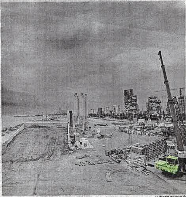
La planta de hormigonado de las obras
